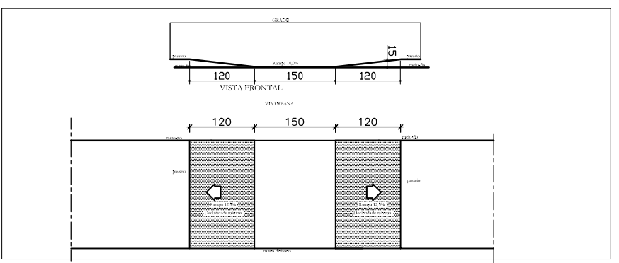
DETALHE DA RAMPA DE PASSEIO
